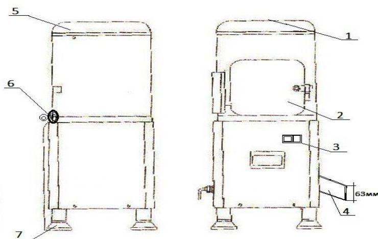
Общий вид картофелечистки ( Рис 1)
